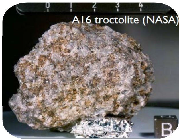
月のトロクトライト（NASA）
