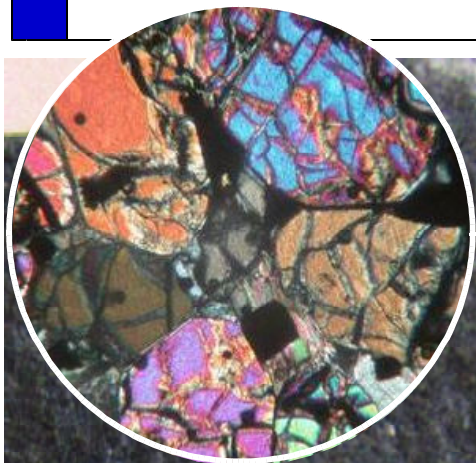
トロクトライトの薄片写真
